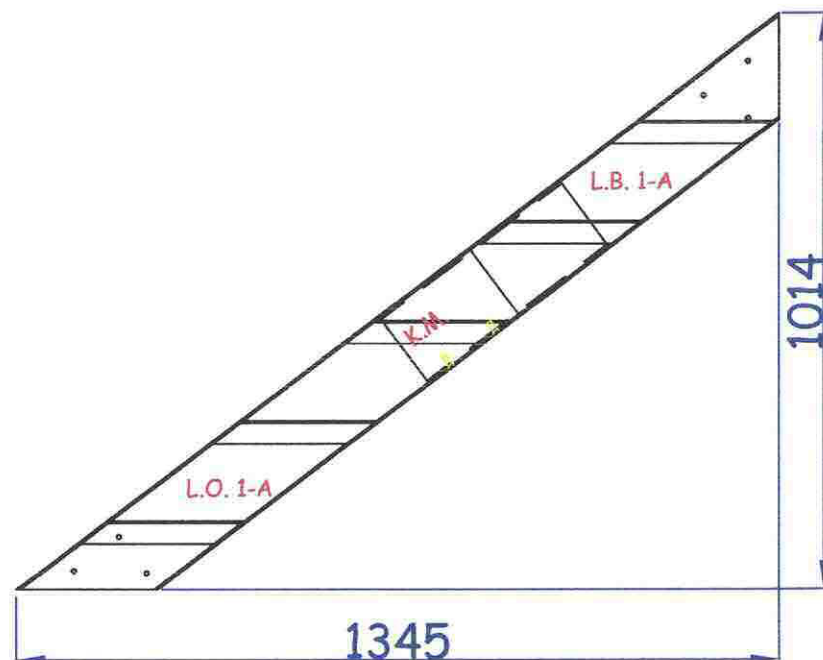
Escalier 5 marches
