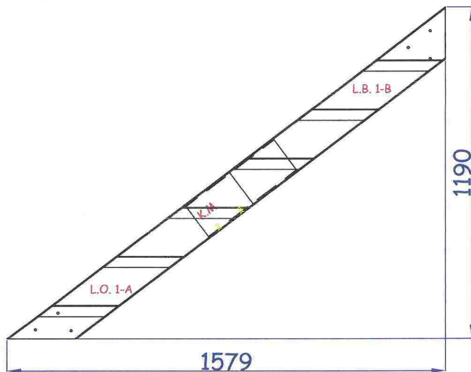
Escalier 6 marches
