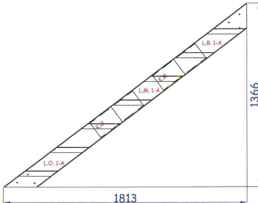
Escalier 7 marches
