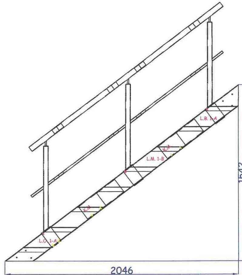
Trap 8 treden Leuning <600-600>
