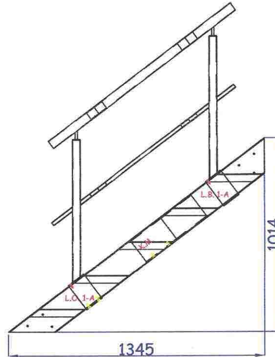
Trap 5 trede Leuning <600>
