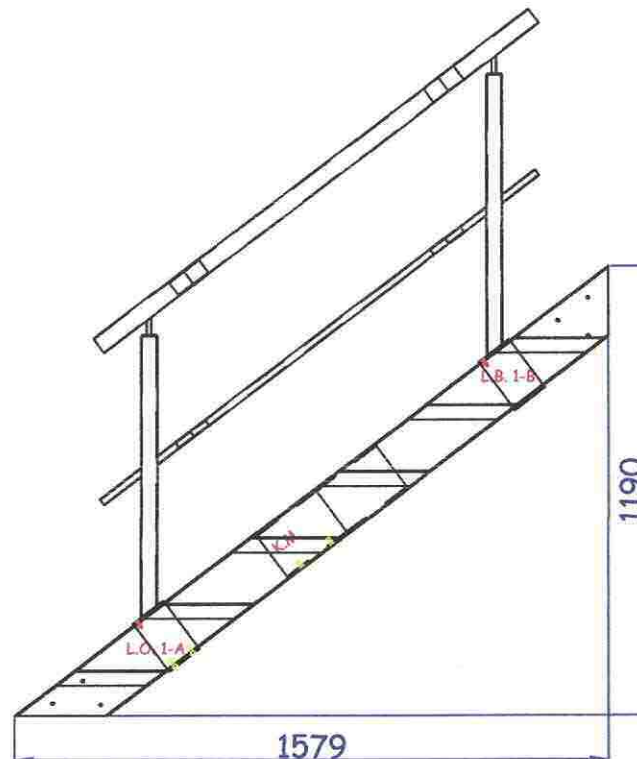
Trap 6 treden Leuning <850>
