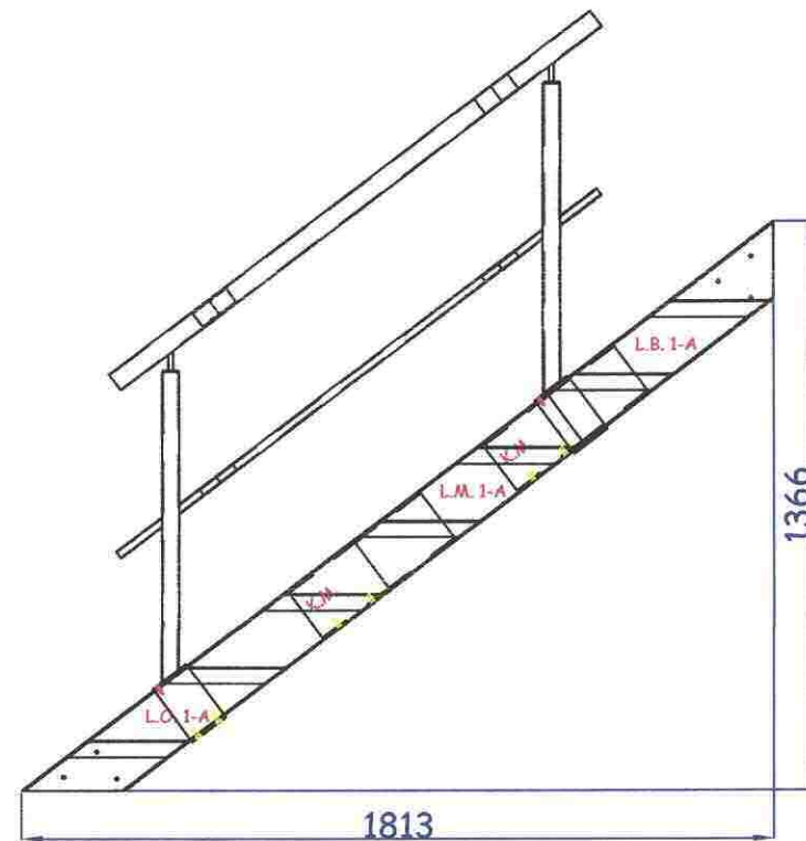
Trap 7 treden Leuning <850>
