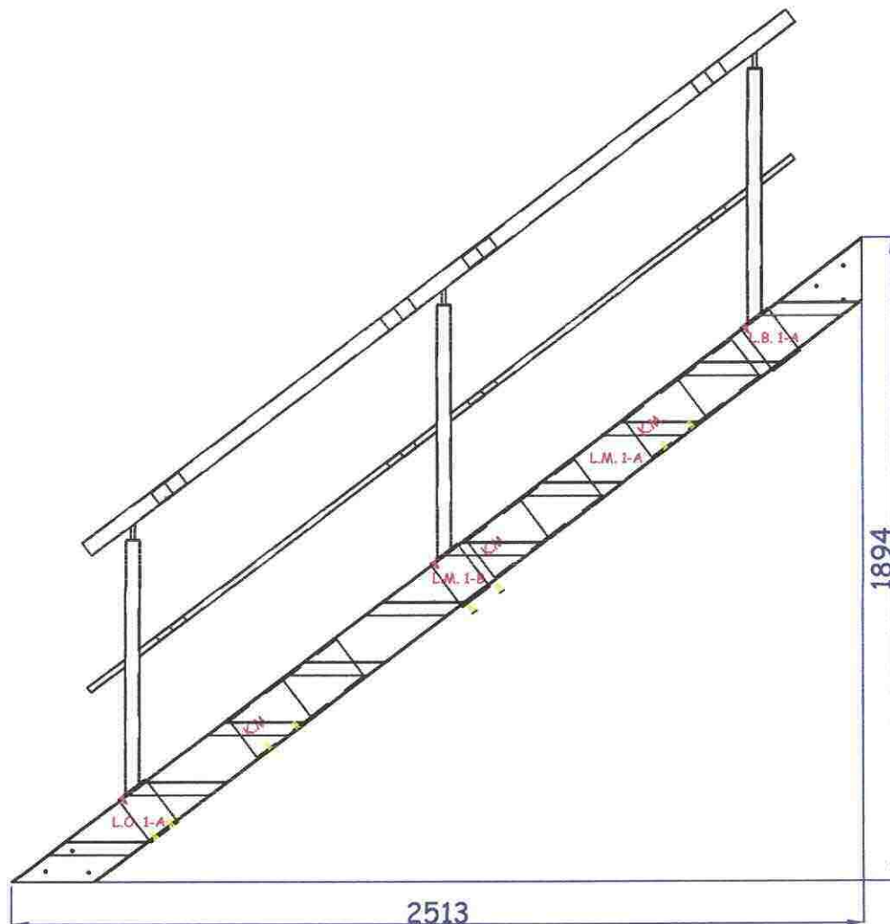
Trap 10 treden Leuning <850-850>
