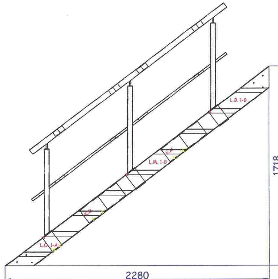
Trap 9 treden Leuning <600-600>
